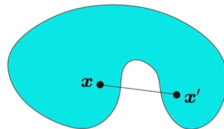
Nonconvex
